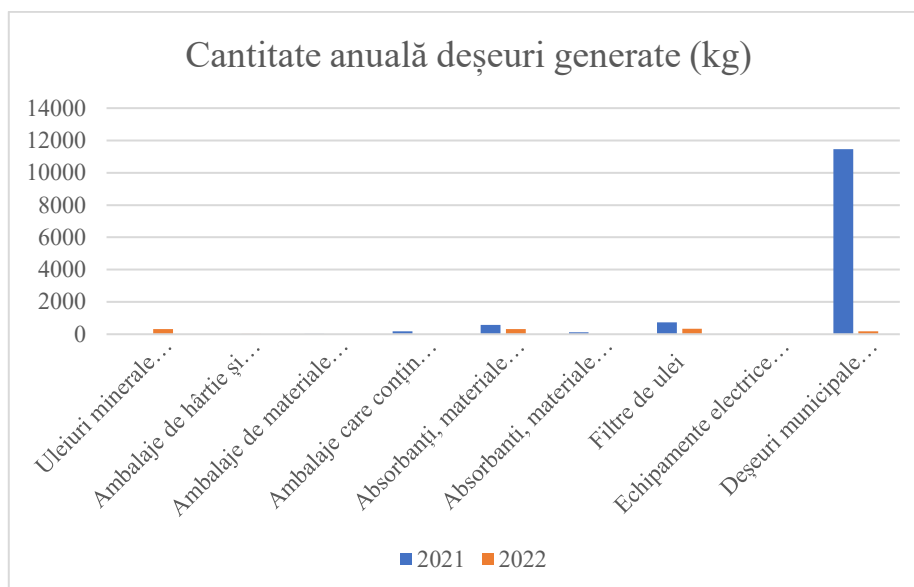
Figura 2: Cantitate (kg) anuală de deșuri generată la nivelul anilor 2021 și 2022 – CEE Vutcani
