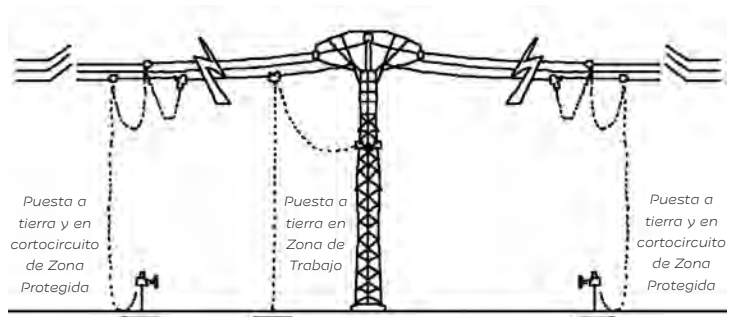
Figura 12. Disposición de las puestas a tierra cuando el trabajo se realice en un solo conductor y se mantengan las distancias suficientes a otros conductores
